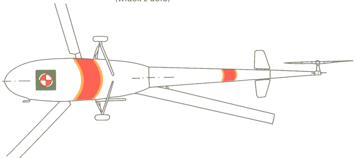
WZÓR OZNAKOWANIA ŚMIGŁOWCA STRAŻY GRANICZNEJ (widok z dołu)
