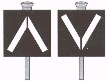
Rys. 176. Wskaźnik W 10a i W 10b
