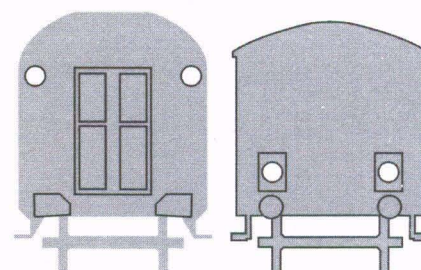
Rys. 136. Sygnał Pc 4 (dzienny i nocny)
