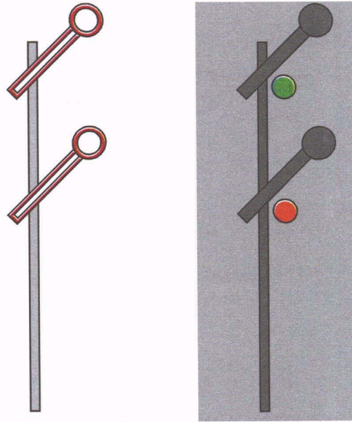
Rys. 3. Sygnał Sr 3
