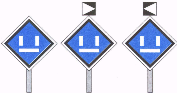
Rys. 203. Wskaźniki We 8a, We 8b, We 8c
