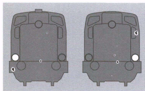
Rys. 139. Sygnał Tb 1 (dzienny i nocny)
