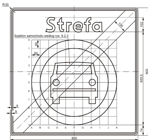
Rys. 9.4.81. Konstrukcja znaku D-55
