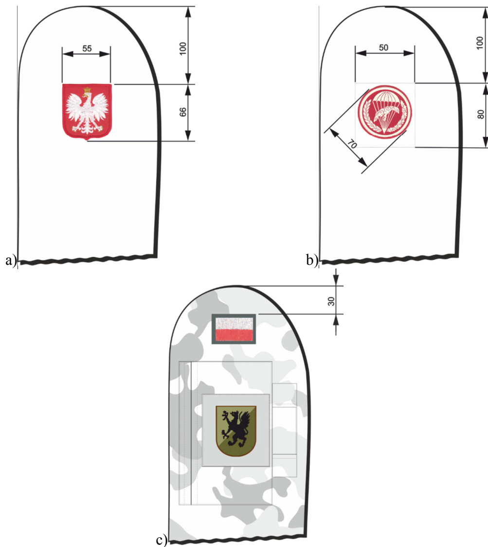
Rys. 1. Sposób rozmieszczenia oznak przynależności państwowej i rozpoznawczych a) oznaka przynależności państwowej - na rękawie kurtki munduru i płaszcza b) oznaka rozpoznawcza – na rękawie kurtki munduru i płaszcza c) oznaka przynależności państwowej i rozpoznawcza na rękawie bluzy polowej
