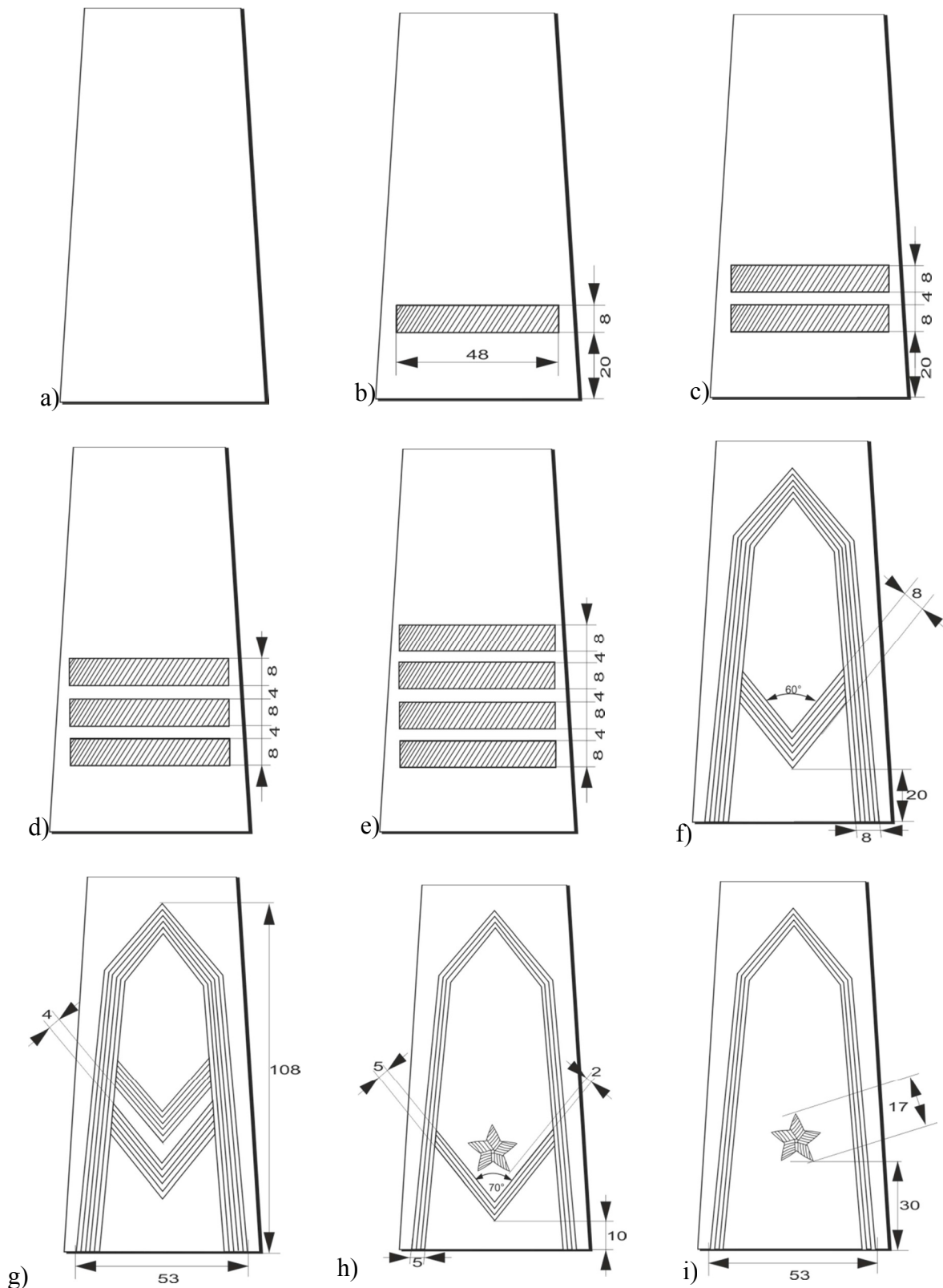
Rys. 9. Sposób rozmieszczania oznak stopni wojskowych na pochewce
