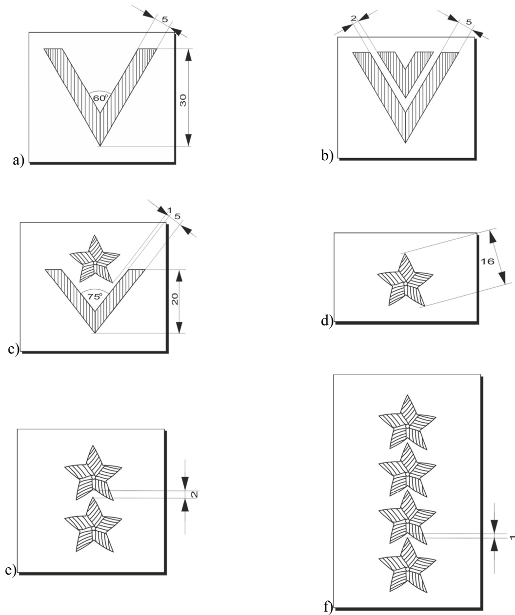
Rys. 10. Sposób rozmieszczenia oznak stopni wojskowych na beretach i furażerkach
