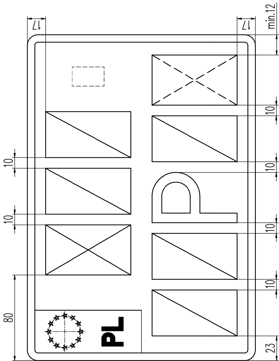
Odmiany profesjonalnych tablic samochodowych dwurzędowych
