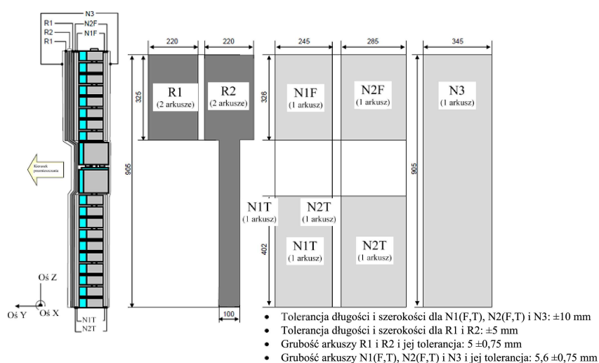
Elastyczny model dolnej części nogi: Wymiary ciała i skóry
