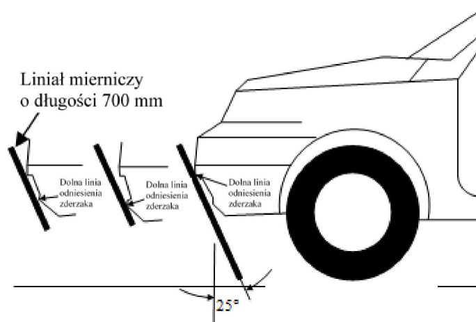
Dolna linia odniesienia zderzaka
