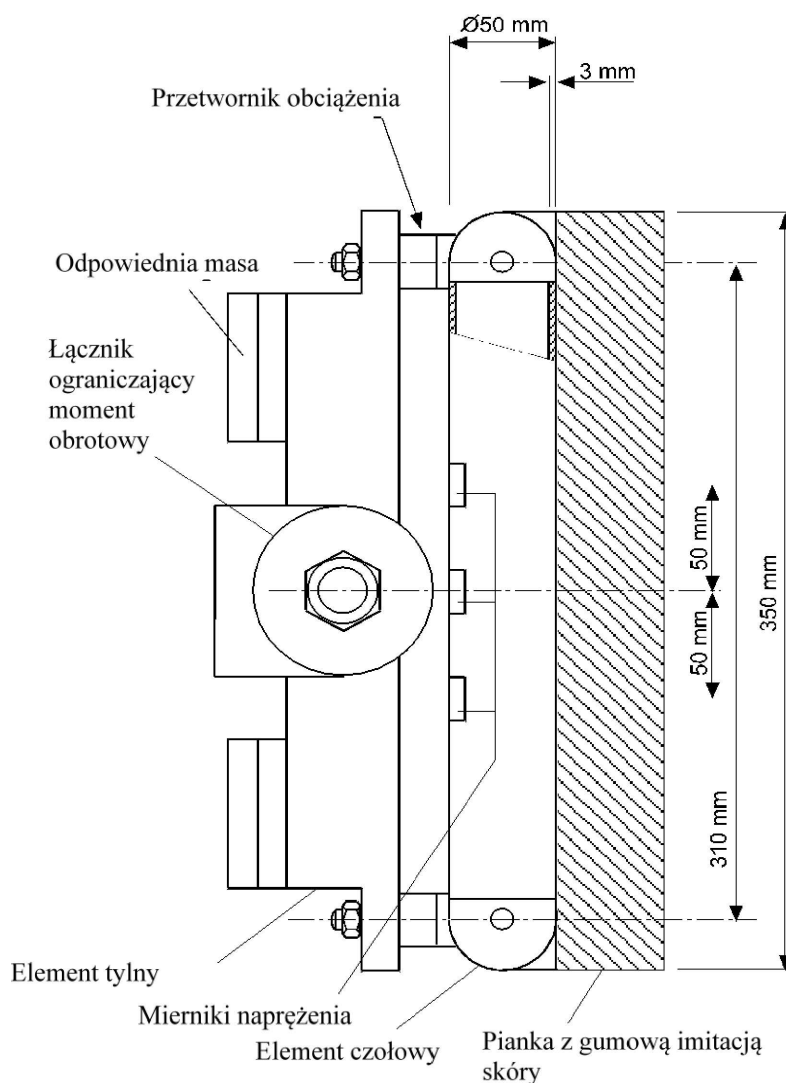
Model górnej części nogi
