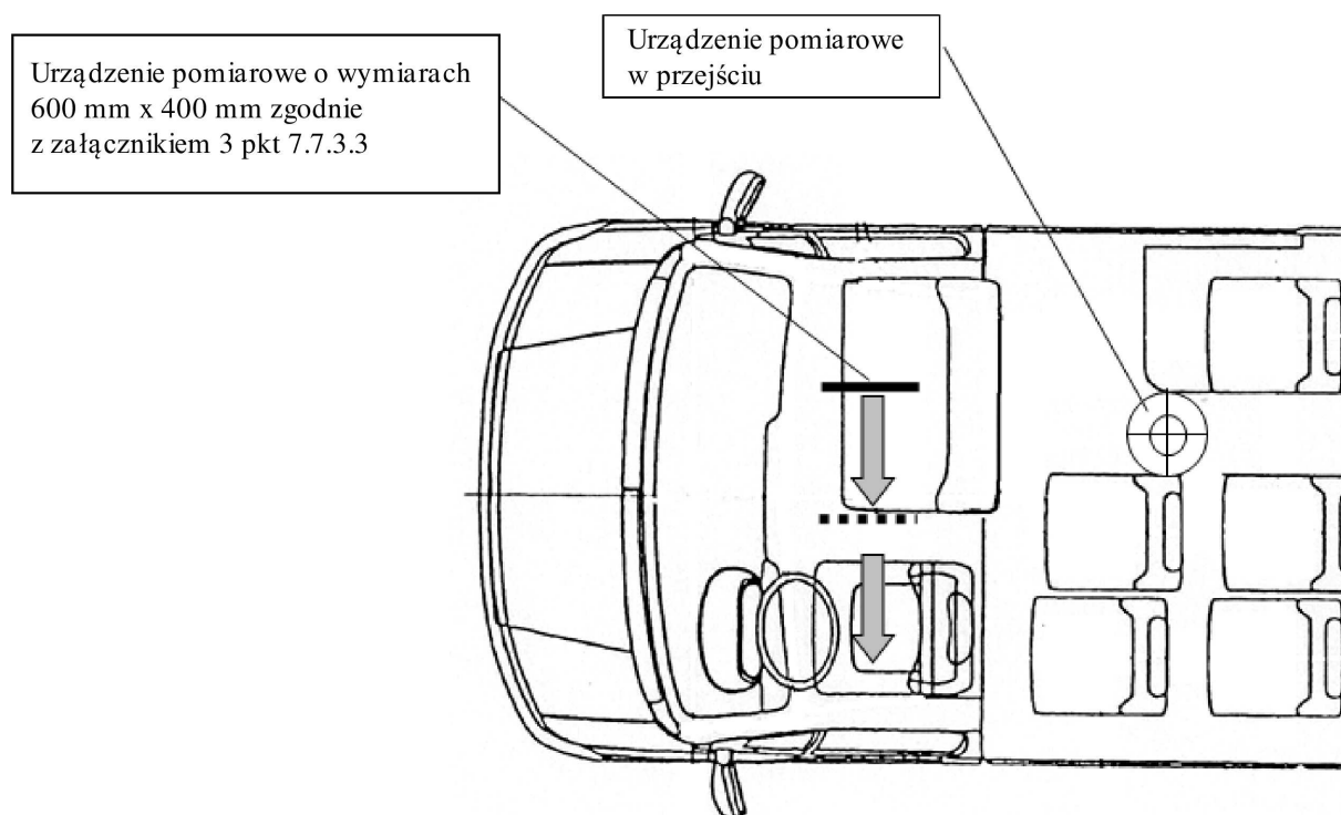
Rysunek 27 Dostęp do drzwi kierowcy (zob. załącznik 3 pkt 7.6.1.7.2)
