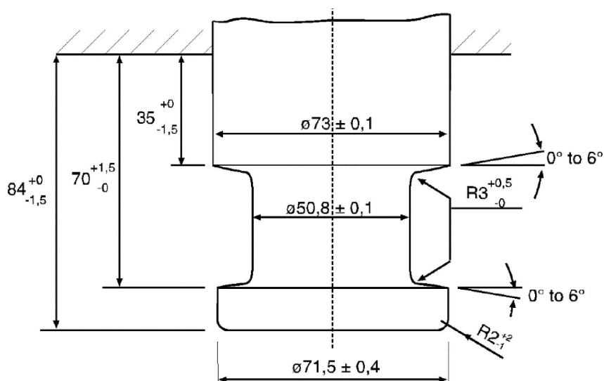
Wymiary sworzni sprzęgu siodłowego klasy H50
