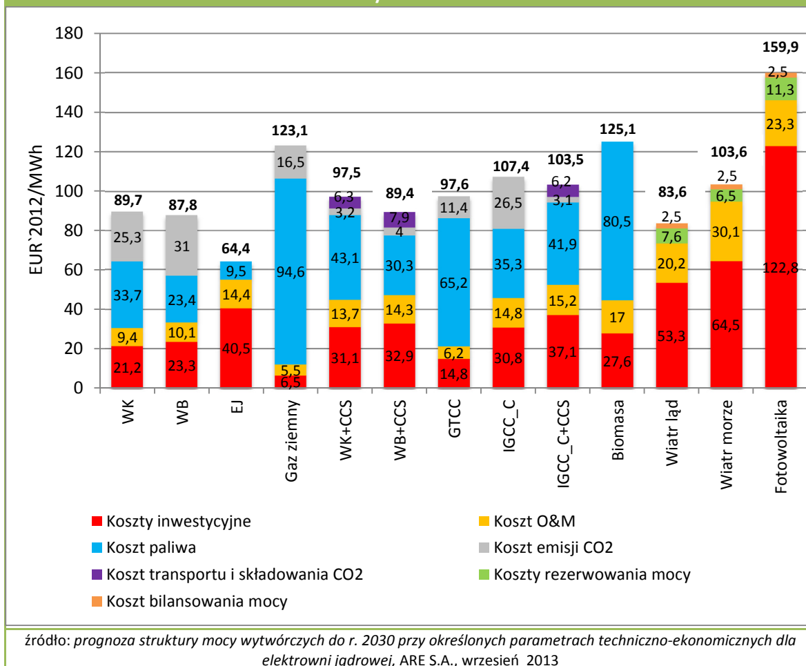
Rys. 4.12.1 Uśredniony jednostkowy koszt wytwarzania energii elektrycznej w źródłach przewidzianych do uruchomienia w 2025 r. przy parametrach dla nowobudowanych źródeł wytwarzania
