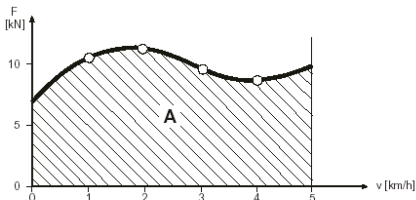
Wzorcowy wykres siły hamowania (Wyznaczanie powierzchni AA i AB )
