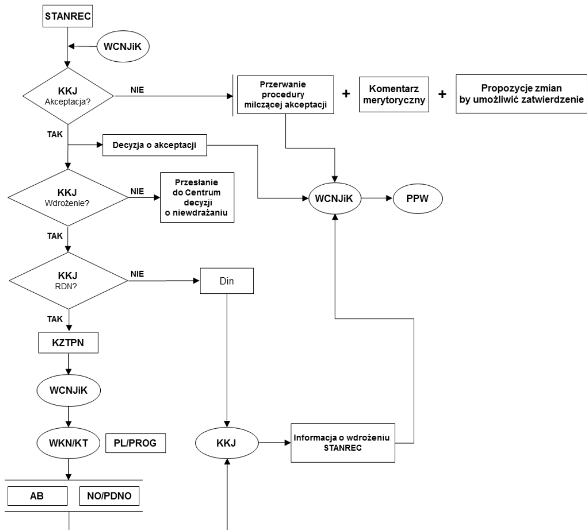
Rysunek 2. Algorytm postępowania z dokumentem STANREC.
