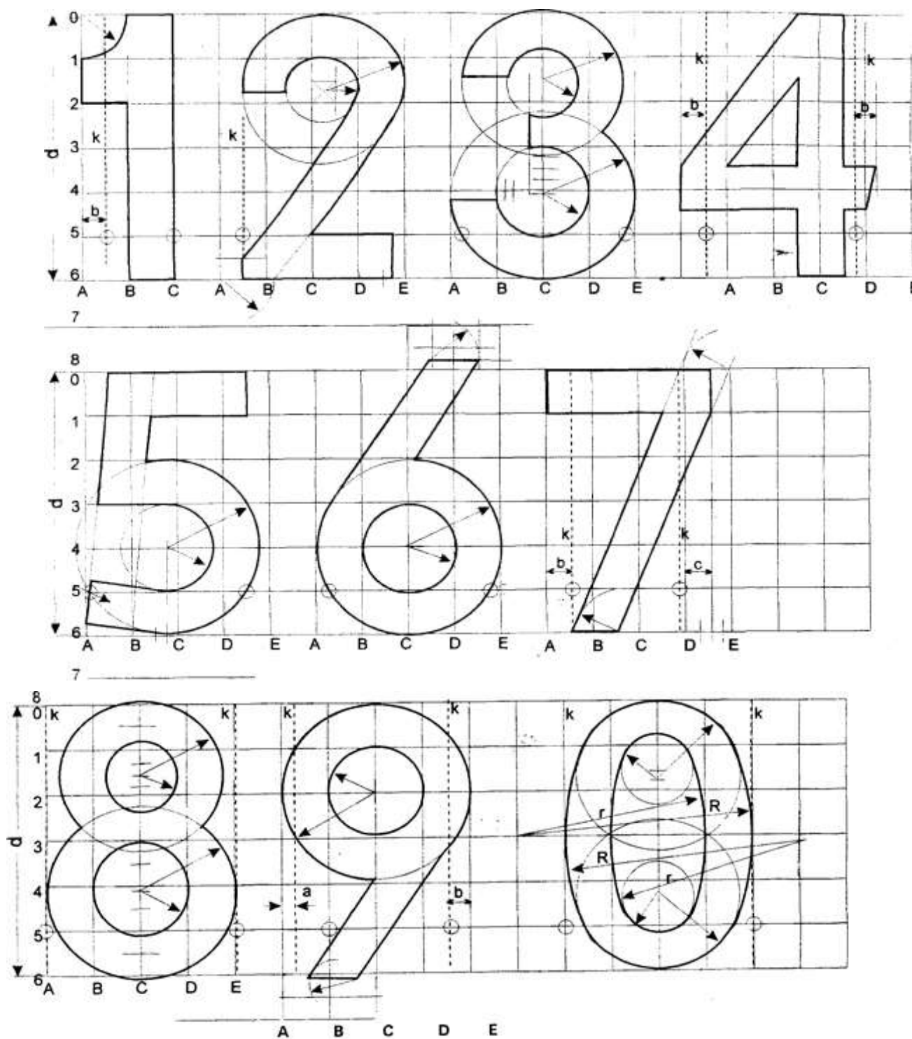
Rysunek. Wzory proporcji liter i cyfr stosowanych w napisie numeru taktycznego
