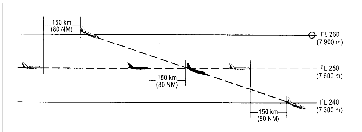
Rysunek 5-26B. Separacja — przy stosowaniu RNAV — 150 km (80 NM) między statkami powietrznymi podczas zniżania na tej samej linii drogi (patrz pkt 5.4.2.5.5. lit. c))
