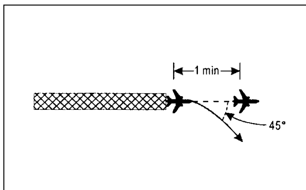
Rysunek 5-35. Separacja jednoczynowa między odlatającymi statkami powietrznymi z kątami drogi różniącymi się nie mniej niż 45° (patrz pkt 5.6.1.)
