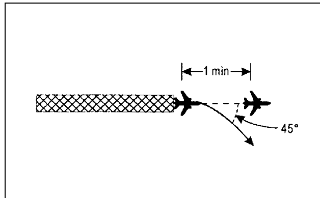
Rysunek 5-37. Separacja jednocminutowa między odlatującymi statkami powietrznymi z kątami drogi różniącymi się nie mniej niż 45° (patrz pkt 5.6.1.)
