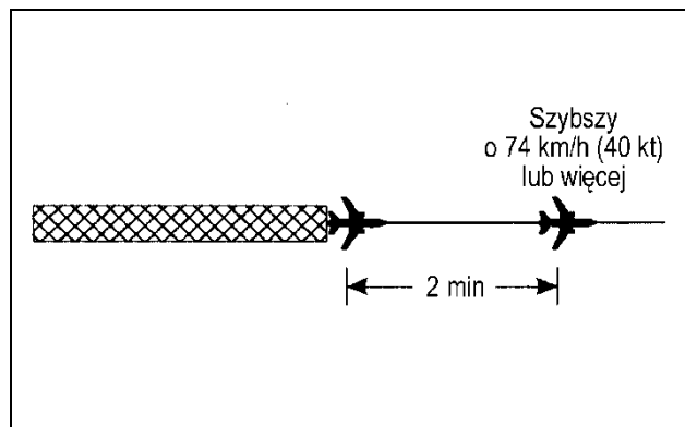
Rysunek 5-38. Separacja dwucminutowa między statkami powietrznymi lecącymi po tej samej linii drogi (patrz pkt 5.6.2.)
