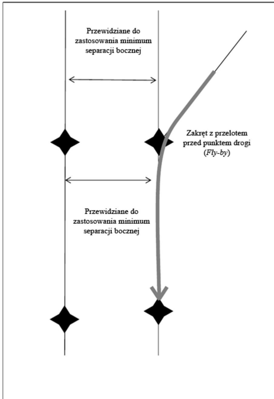
Rysunek 5-2. Zakręt z przelotem przed punktem drogi (patrz pkt. 5.4.1.1.4)
