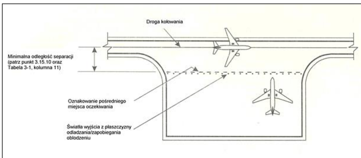
Rysunek 5-28. Przykład oddalonego stanowiska do odladania / przeciwdziałania oblodzeniu
