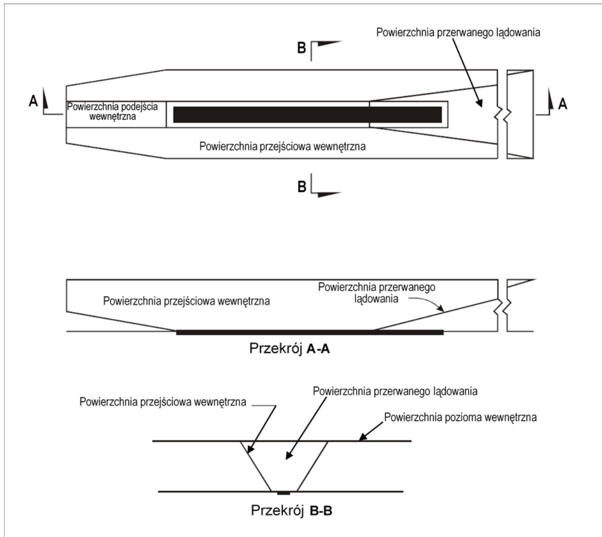
Rysunek 4-2. Powierzchnie ograniczające przeszkody: powierzchnia podejścia wewnętrzna, przejściowa wewnętrzna i przerwane lądowania.
