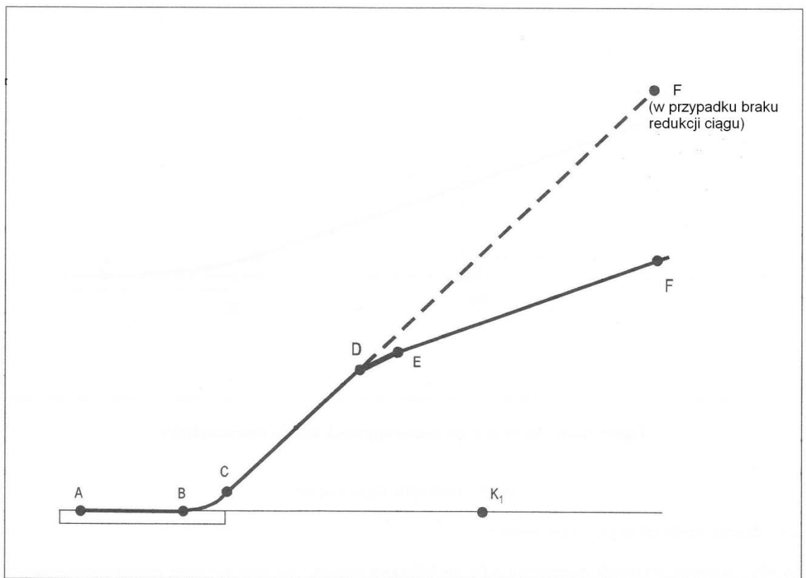
Rys. A2-5. Charakterystyki wzorcowego profilu dla samolotu przy przelocie
