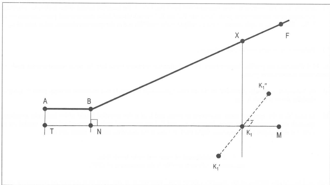
Rys. A2-7. Charakterystyki wzorcowego profilu dla startu samolotu
