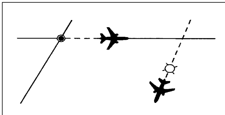
Rysunek 5-3. Korzystanie z tych samych lub różnych punktów geograficznych (patrz pkt 5.4.1.2.1.1)
