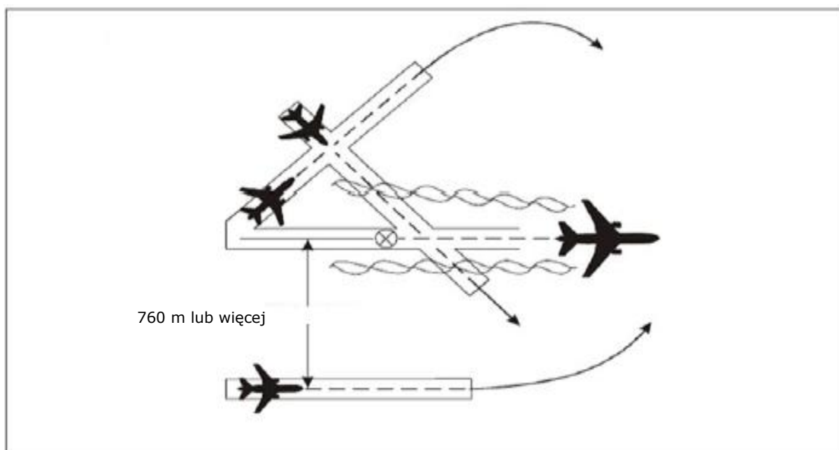
Rysunek 5-43. Separacja dla statków powietrznych, których linie drogi przecinają się, w warunkach turbulencji w śladzie aerodynamicznym (patrz pkt 5.8.3.1. lit c) i d) i pkt 5.8.3.2 lit c) i d))
