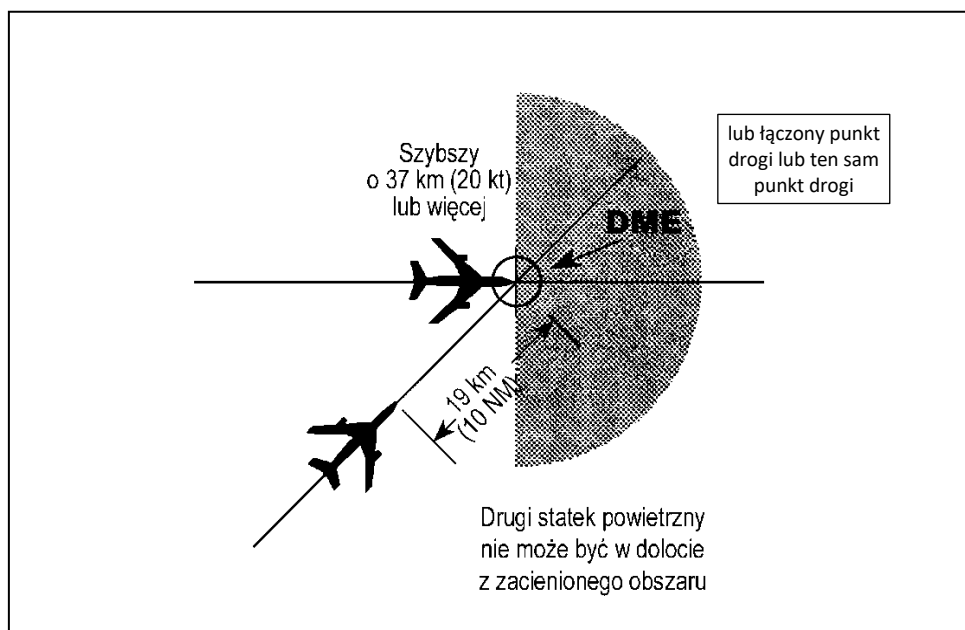
Rysunek 5-24B. Separacja — przy wykorzystaniu DME lub GNSS — 19 km (10 NM) między statkami powietrznymi na przecinających się liniach drogi i na tym samym poziomie lotu (patrz pkt 5.4.2.3.3.2)
