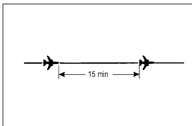
Rysunek 5-10. Separacja piętnastominutowa między statkami powietrznymi na tej samej linii drogi i na tym samym poziomie lotu (patrz pkt 5.4.2.2.1.1 lit. a))
