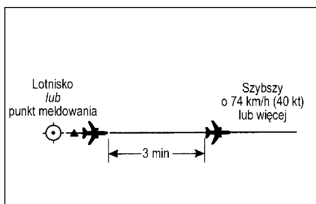
Rysunek 5-13. Separacja trzuminutowa między statkami powietrznymi na tej samej linii drogi i na tym samym poziomie lotu (patrz pkt 5.4.2.2.1.1 lit. d))
