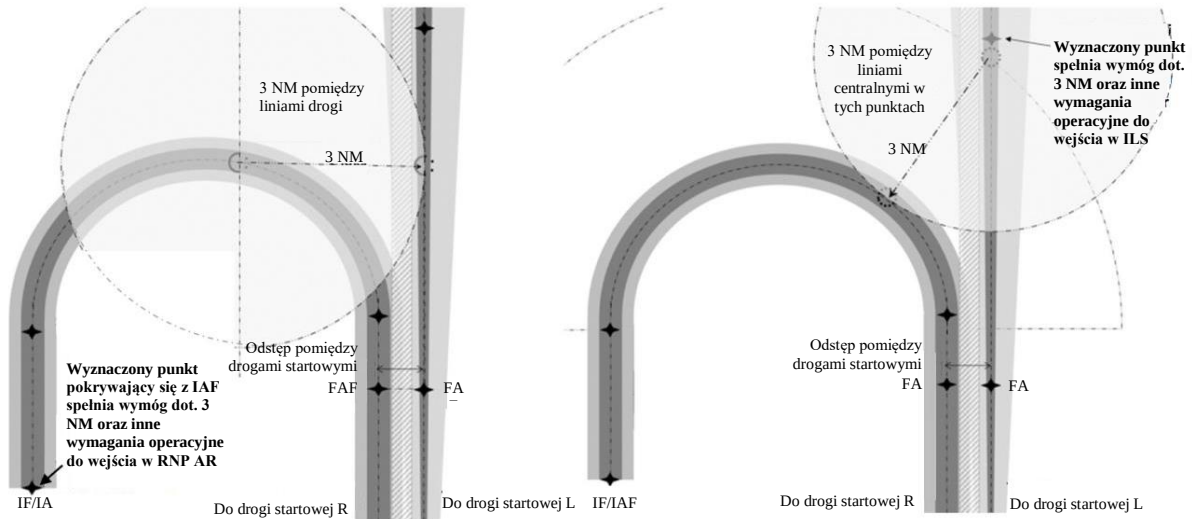
Rysunek 6-6. Koncepcja „ustabilizowania na RNP AR APCH” (RNP AR APCH/Podejście precyzyjne z przykładem minimalnej separacji 3NM)
