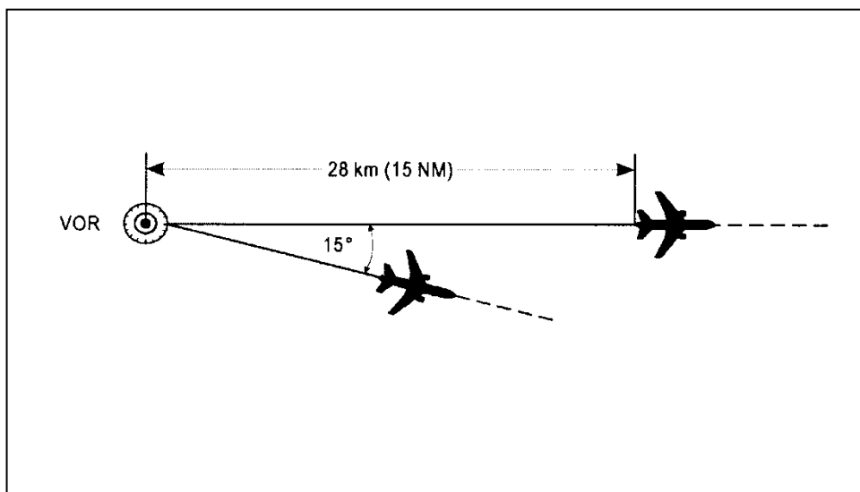
Rysunek 5-3. Korzystanie z tych samych lub różnych punktów geograficznych (patrz pkt 5.4.1.2.1.1)
