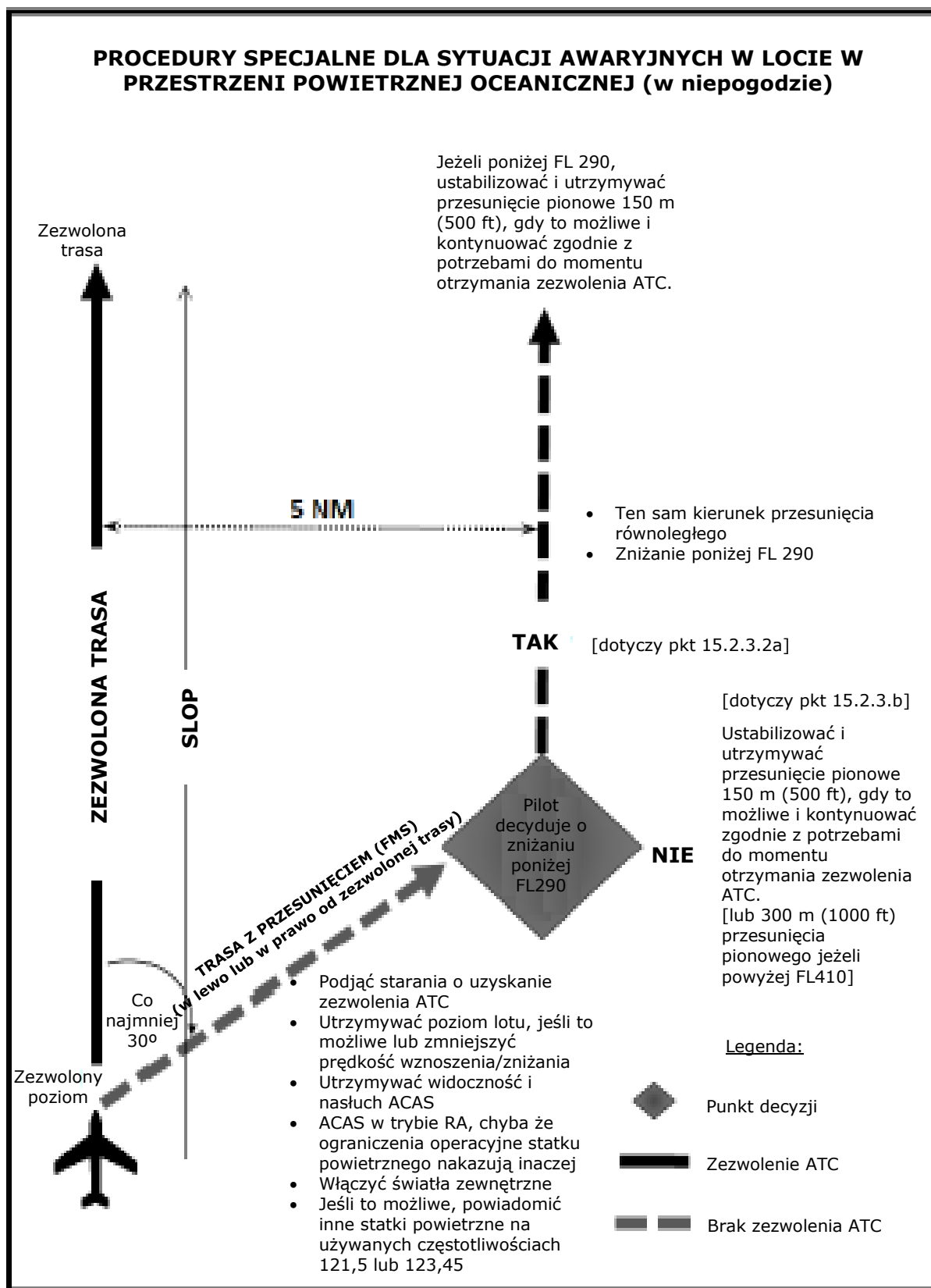
Rysunek 15-1. Prowadzenie wzrokowe w procedurach w sytuacji awaryjnej (patrz 15.2.2 i 15.2.3)
