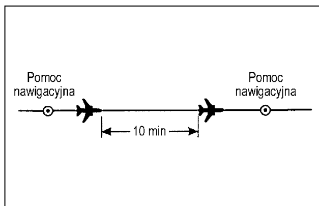
Rysunek 5-11. Separacja dziesięciominutowa między statkami powietrznymi na tej samej linii drogi i na tym samym poziomie lotu (patrz pkt 5.4.2.2.1.1 lit. b))
