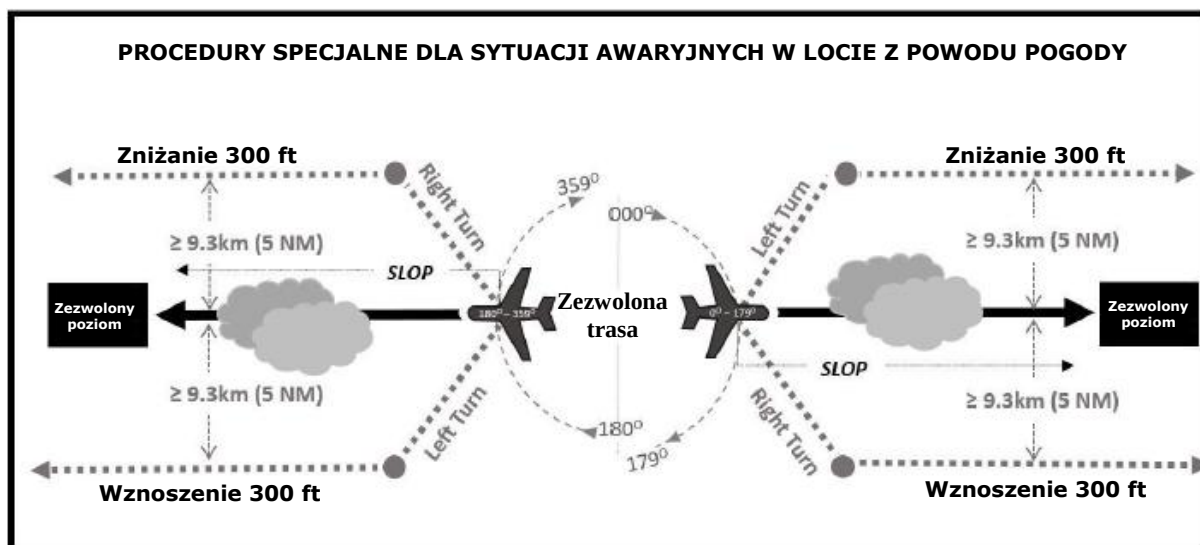
Rysunek 15-2. Prowadzenie wzrokowe w przypadku procedur odchylenia od trasy z powodu pogody, gdy zmienione zezwolenie ATC nie może być otrzymane (patrz pkt 15.2.4.3)
