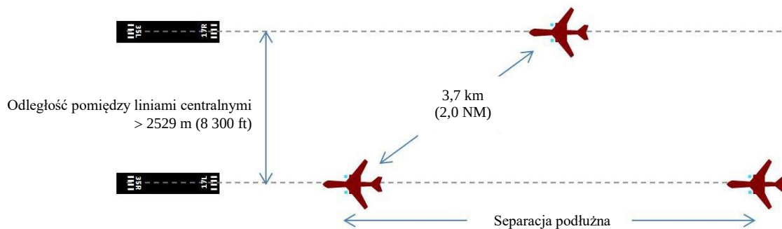
Rysunek 6-3. Separacja przekątna dla odległości linii centralnych większej niż 2 529 m (8 300 ft)
