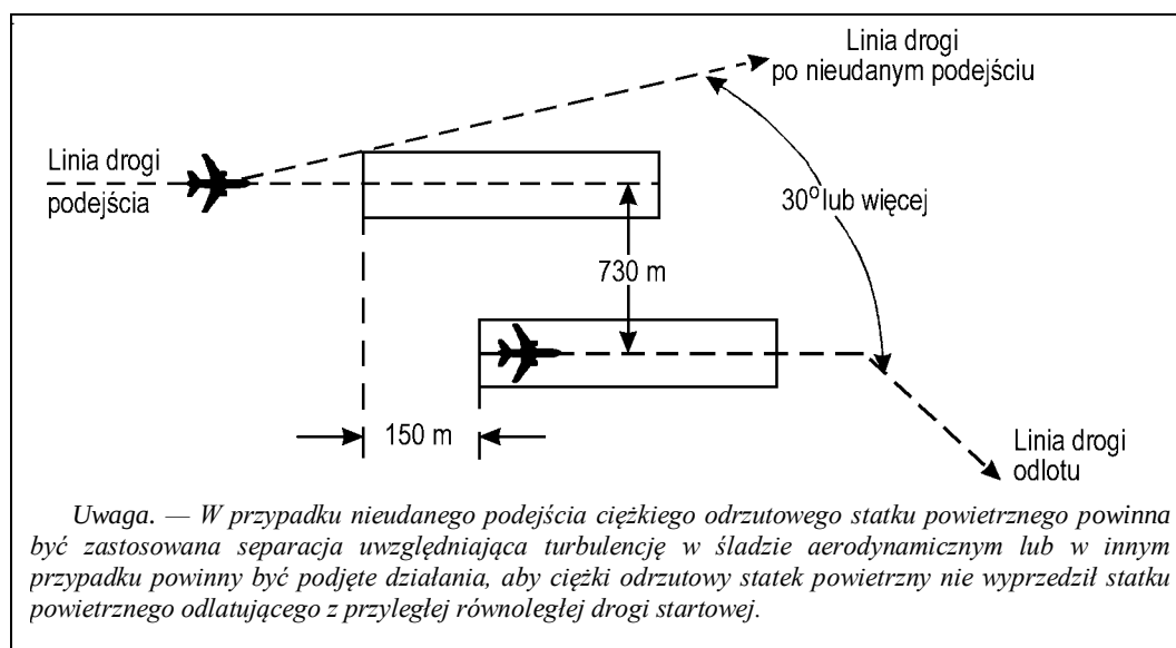
Rysunek 6-8. Rozdzielone operacje równoległe na przesuniętych drogach startowych (patrz pkt 6.7.3. 6.2)
