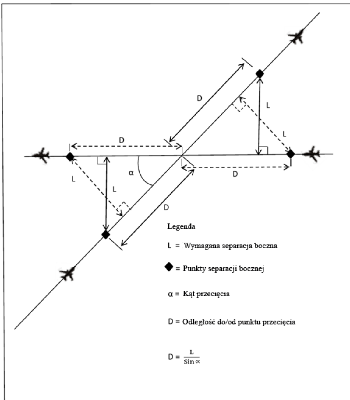
Rysunek 5-6. Punkty separacji bocznej (patrz pkt 5.4.1.2.1.7)
