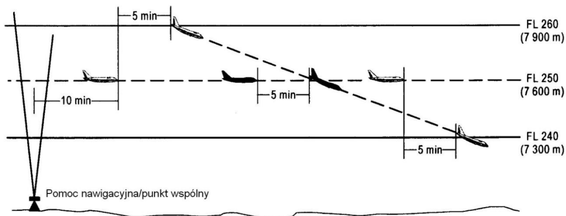
Rysunek 5-18B. Separacja pięciominutowa między statkami powietrznymi podczas zniżania i na tej samej linii drogi (patrz pkt 5.4.2.2.2.1 lit. c)2)
