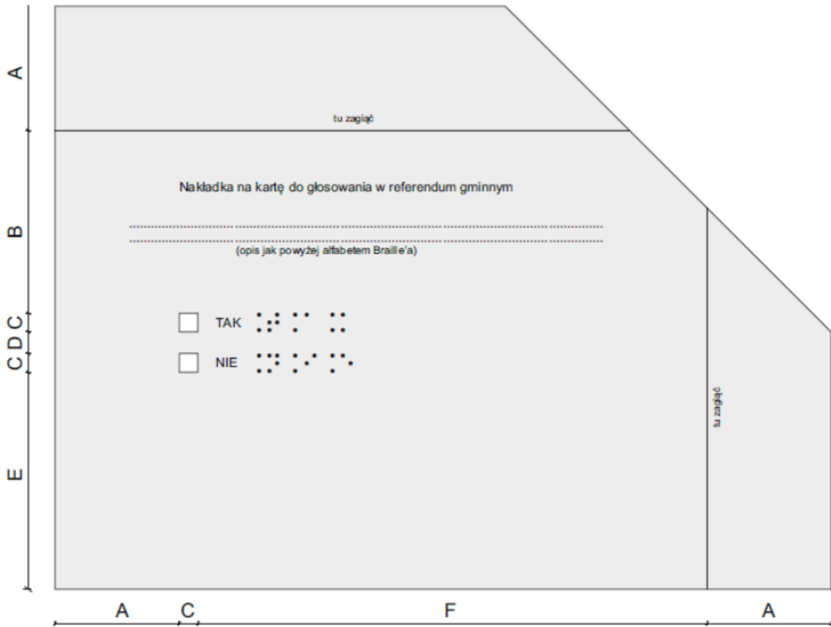
Nakładka formatu A5. A=40 mm, B=59 mm, C=6 mm, D=7 mm, E=70 mm, F=164 mm
