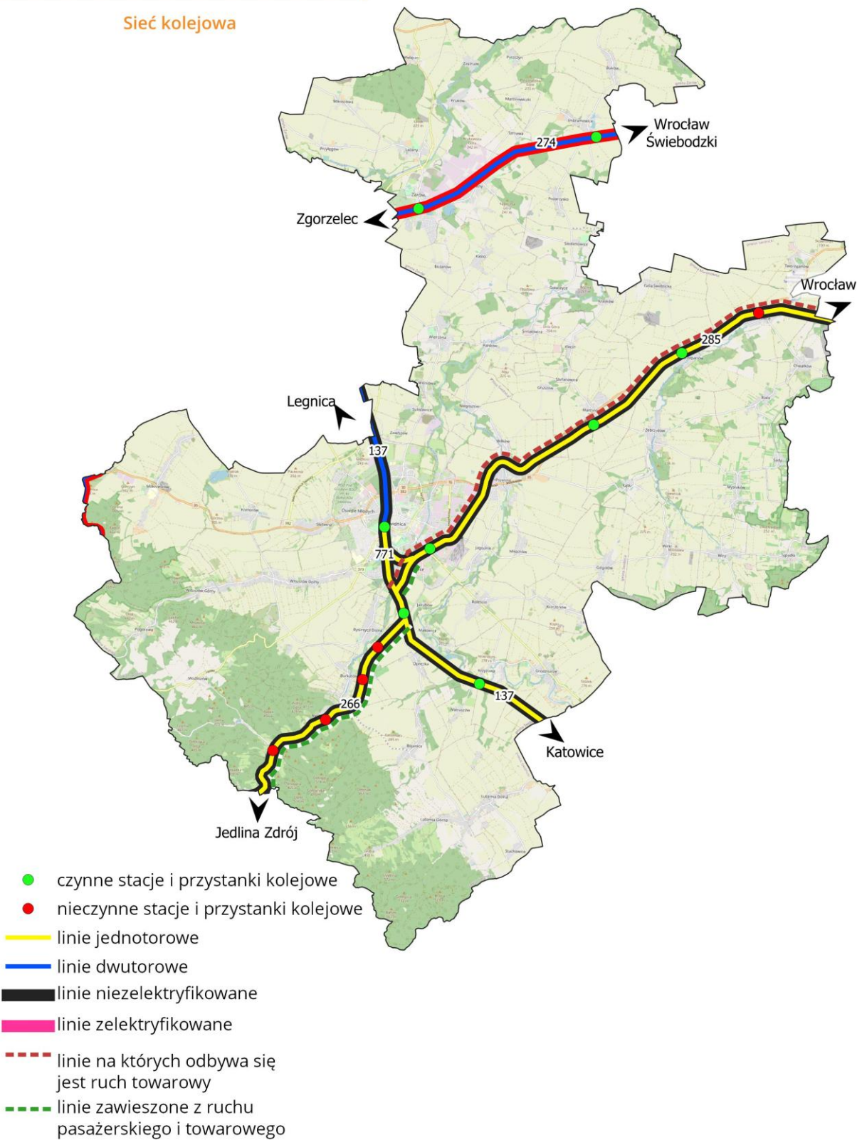
Rys. 4.7 Układ linii kolejowych w okolicach Świdnicy Źródło: Opracowanie własne
