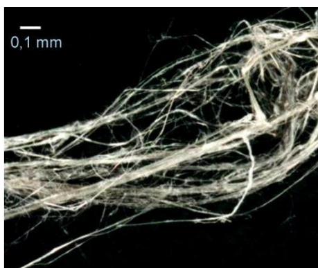
Rys. 1. Długowłókniasty azbest chryzotylowy praktycznie niezawierający zanieczyszczeń (Chiny)
