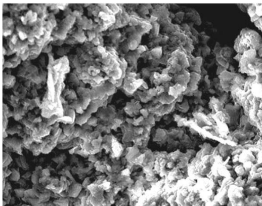
Rys. 3. Erozja płyt a-c – płyty KARO - widoczne pod mikroskopem włókna azbestu (pow. 1000x) (wg J. Dyczek)
