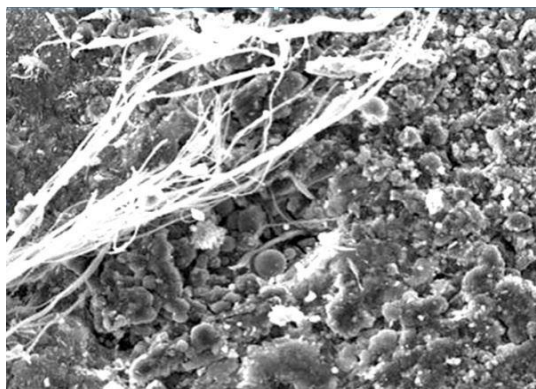
Rys. 4. Erozja płyt a-c – widoczna wiązka całkowicie odsłoniętych włókien (pow. 400x) (wg J. Dyczek)
