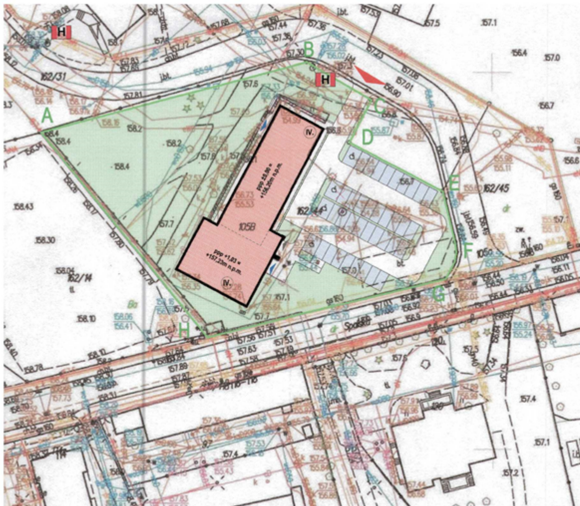
KONCEPCJA ZAGOSPODAROWANIA TERENU INWESTYCJI skala 1:1000
