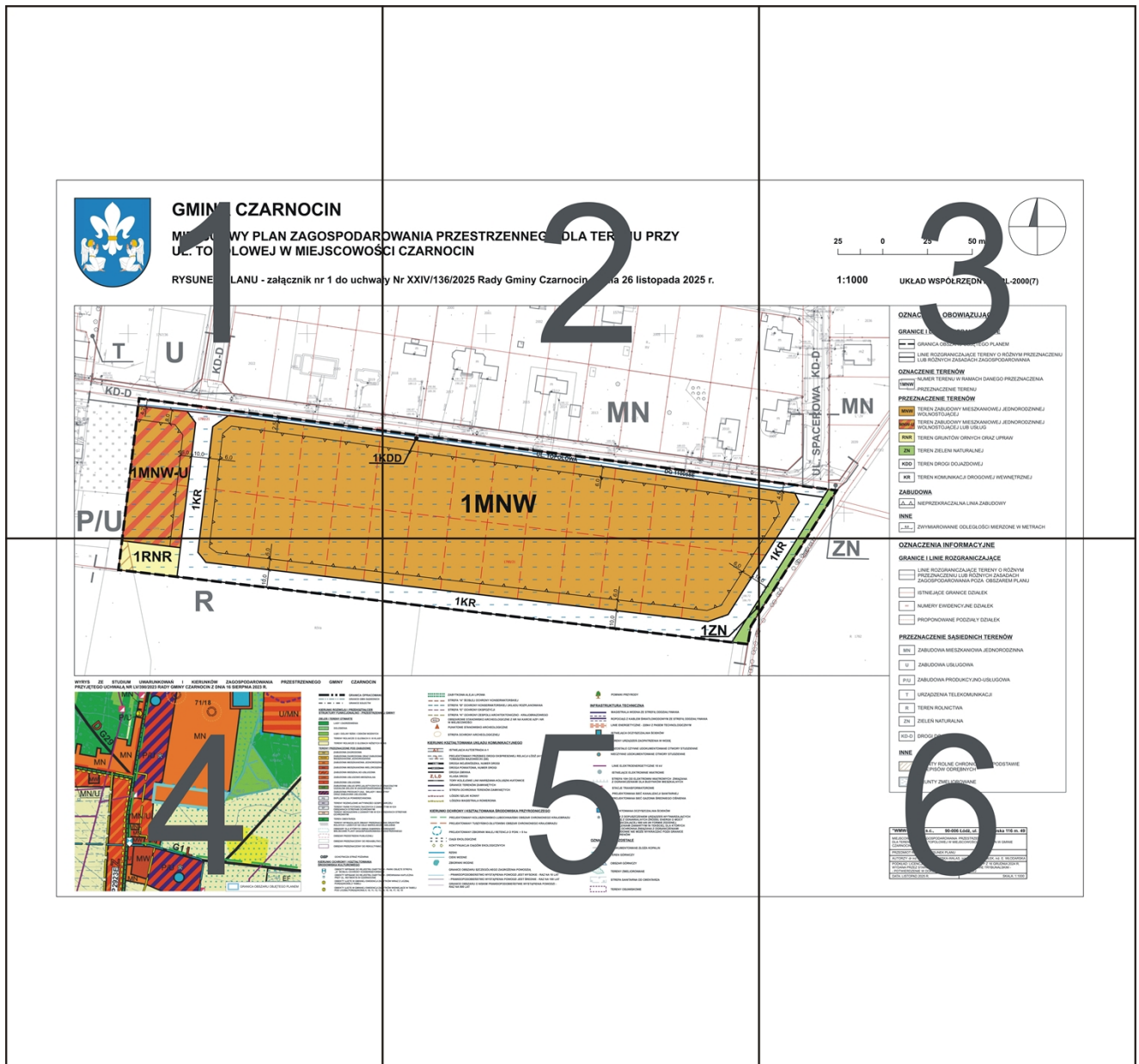
Rysunek planu 1:1000
