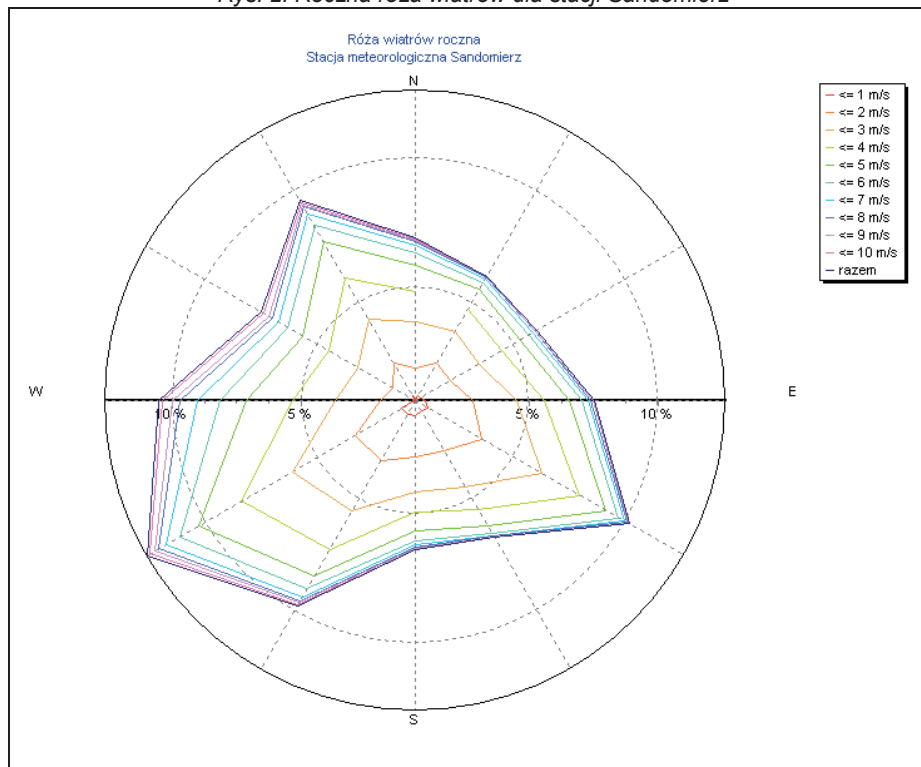
Rys. 2. Roczna róża wiatrów dla stacji Sandomierz
