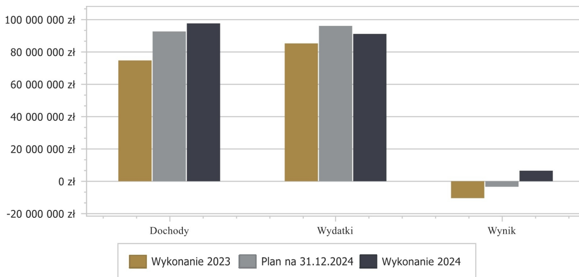
Wykres 1: Wynik budżetu Gminy Mońki w 2024 roku w porównaniu do roku 2023.
