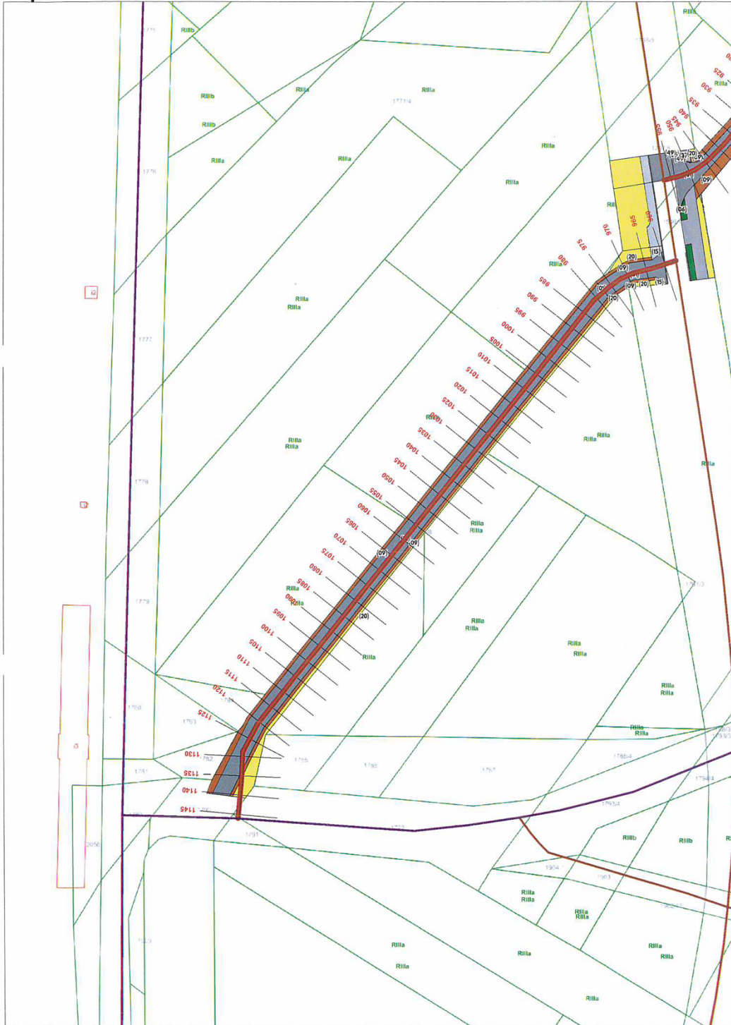
Wydruk wygenerowany za pomocą programu RoadMan (1:1000)
