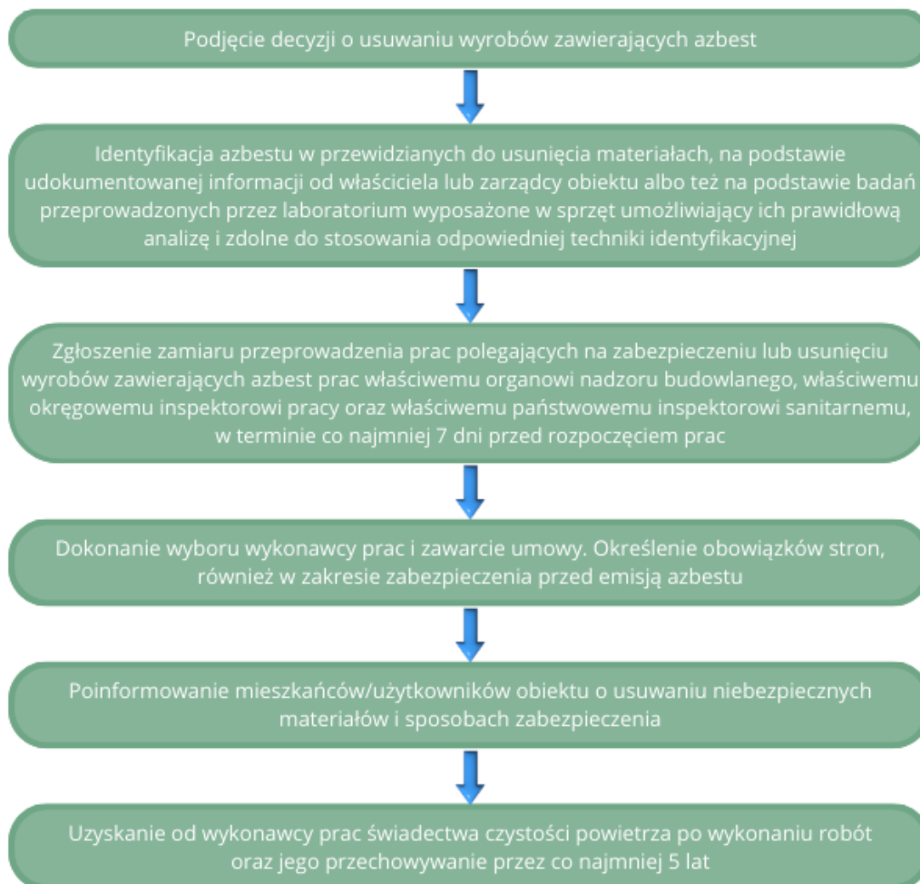
Rysunek 3. Schemat procedury dotyczącej obowiązków i postępowania właścicieli i zarządców przy usuwaniu wyrobów zawierających azbest z obiektów i terenów zlokalizowanych na terenie Gminy Szaflary.
