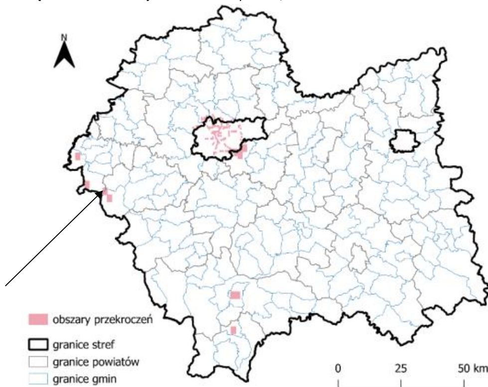
Rysunek 4. Zasięg obszarów przekroczeń dobowego poziomu dopuszczalnego pyłu zawieszonego PM10, określonego ze względu na ochronę zdrowia ludzi w województwie małopolskim, w 2024 roku.
