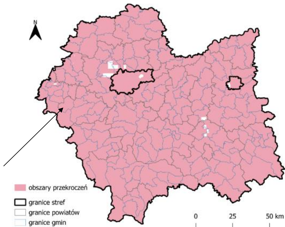
Rysunek 5. Zasięg obszarów przekroczeń poziomu celu długoterminowego dla O 3 , określonego ze względu na ochronę zdrowia ludzi, w województwie małopolskim, w 2024 roku.
