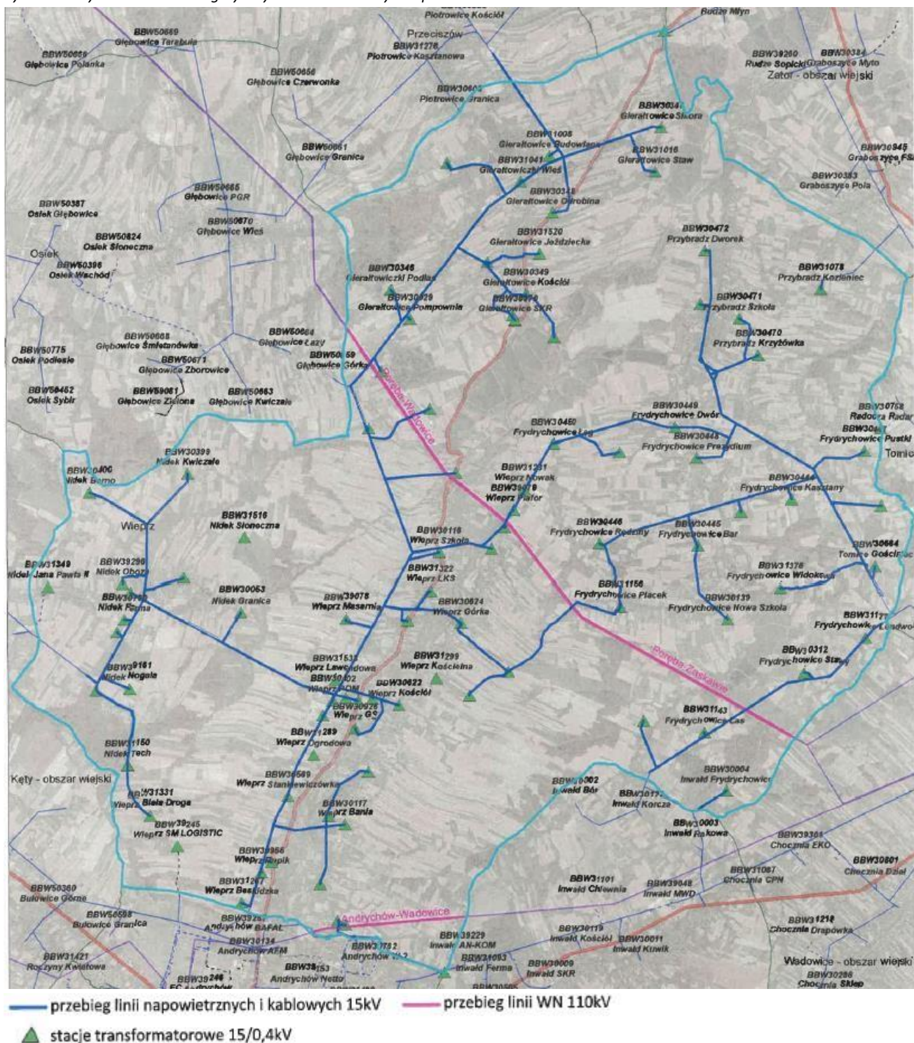
Rysunek 6. System elektroenergetyczny na terenie Gminy Wieprz.
