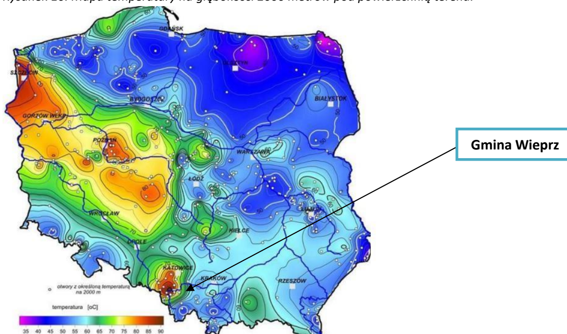
Rysunek 10. Mapa temperatury na głębokości 2000 metrów pod powierzchnią terenu.
