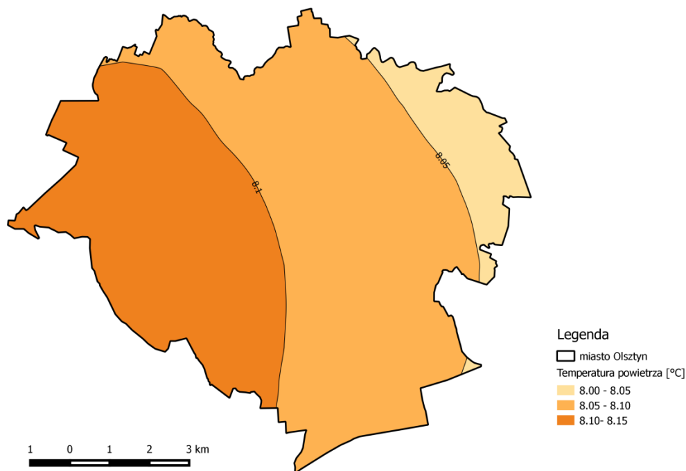
Rysunek 12. Rozkład średniej rocznej temperatury powietrza w strefie miasto Olsztyn w 2014 r.
