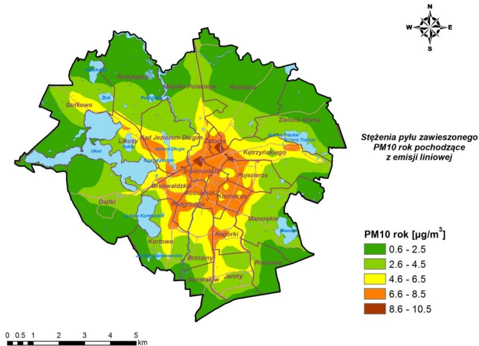
Rysunek 37. Stężenia pyłu zawieszonego PM10 o okresie uśredniania wyników rok w strefie miasto Olsztyn pochodzące z emisji liniowej w 2014 r.
