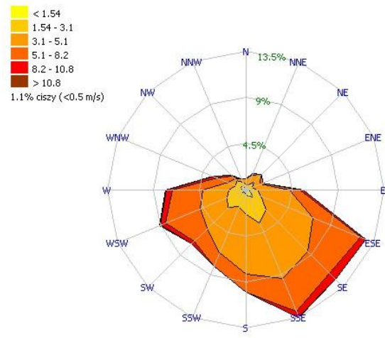
Rysunek 11. Róża wiatrów dla strefy miasto Olsztyn – sezon zimowy w 2014 r.
