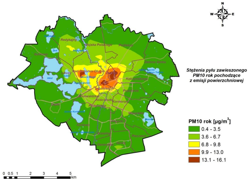
Rysunek 35. Stężenia pyłu zawieszonego PM10 o okresie uśredniania wyników rok w strefie miasto Olsztyn pochodzące z emisji powierzchniowej w 2014 r.
