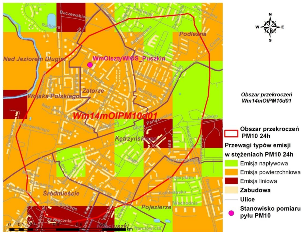
Rysunek 41. Przewagi typów emisji w stężeniach pyłu zawieszonego PM10 24h w obszarze przekroczeń Wm14mOIPM10d01 w strefie miasto Olsztyn w 2014 r.
