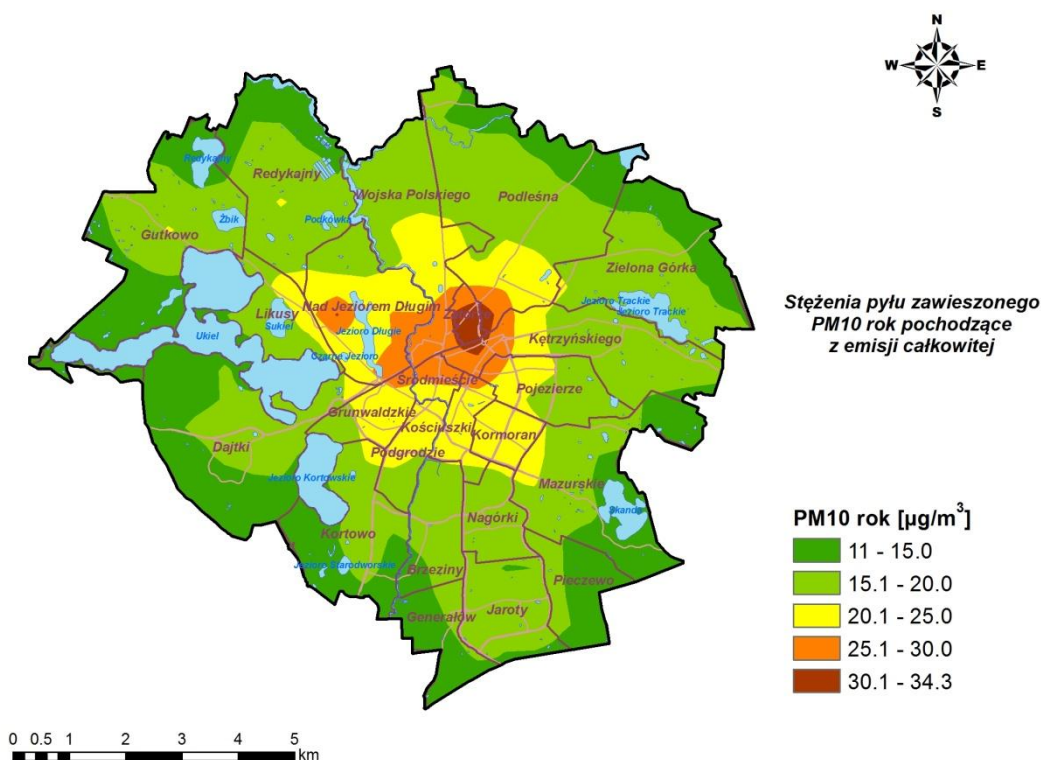
Rysunek 39. Stężenia pyłu zawieszonego PM10 o okresie uśredniania wyników rok w strefie miasta Olsztyn, pochodzące z łącznej emisji wszystkich typów, w 2014 r.
