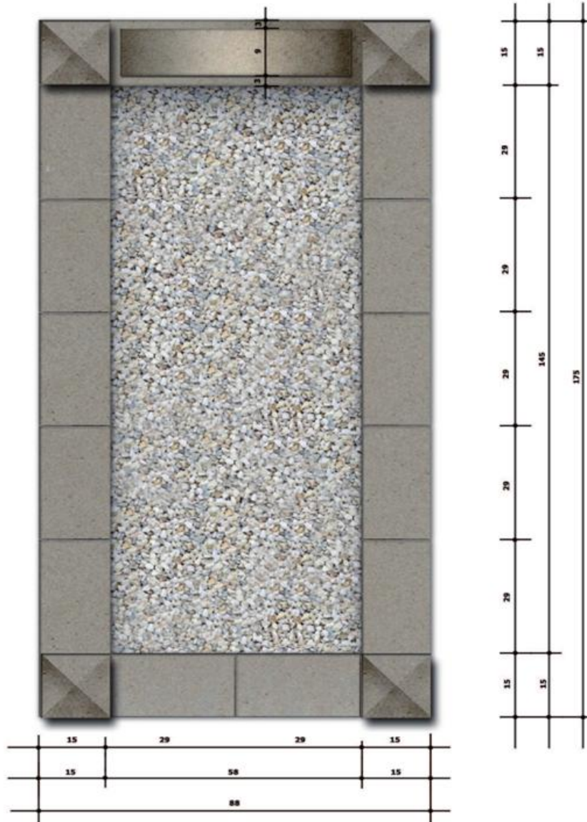
Wymiary pojedynczego nagrobka ogólne wymiary 88 x 175 cm stosować w przypadku, gdy zastane nagrobki w bezpośrednim sąsiedztwie będą miały podobną długość
