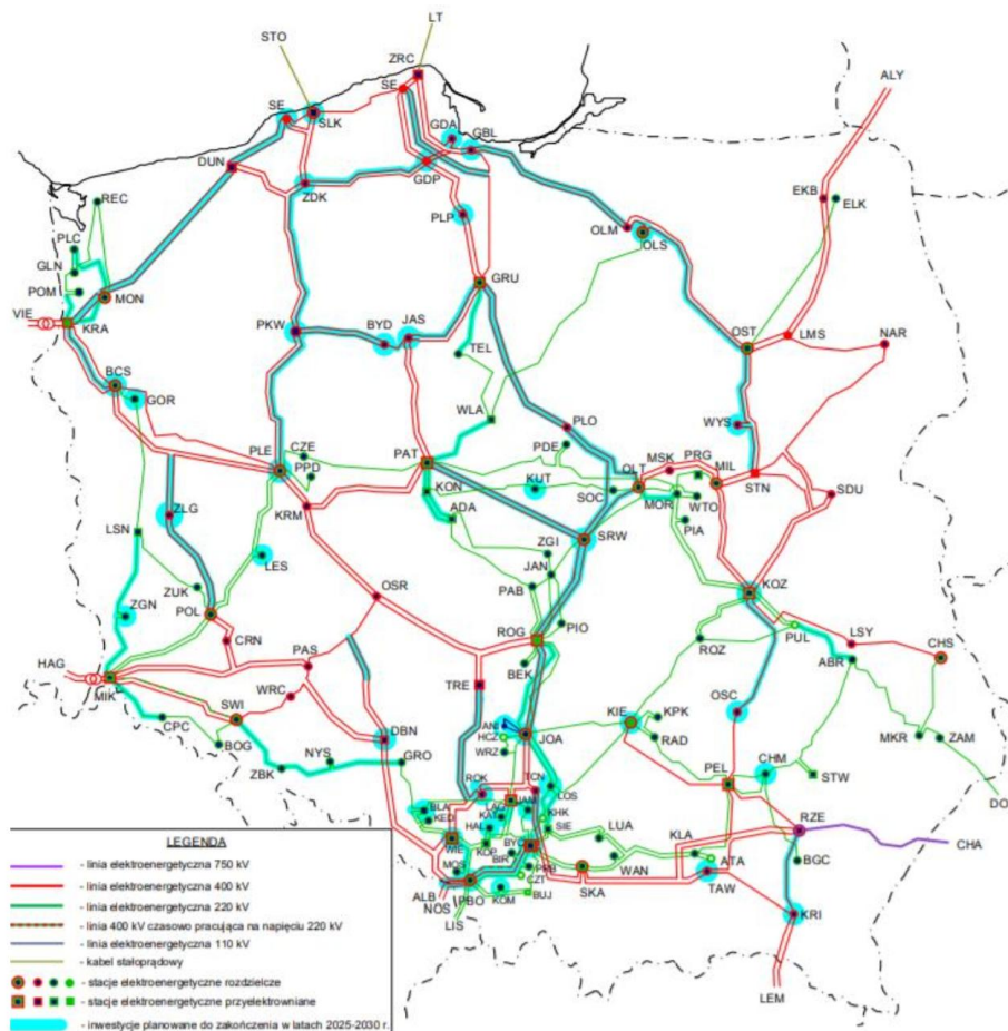
Rycina 19. Schemat sieci przesyłowej 400 i 220 kV – inwestycje planowane do zakończenia do końca roku 2030
