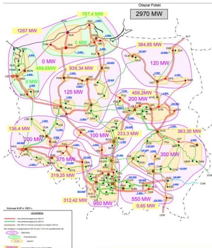
Rycina 18. Schemat sieci przesyłowej z dostępnymi mocami przyłączeniowymi
