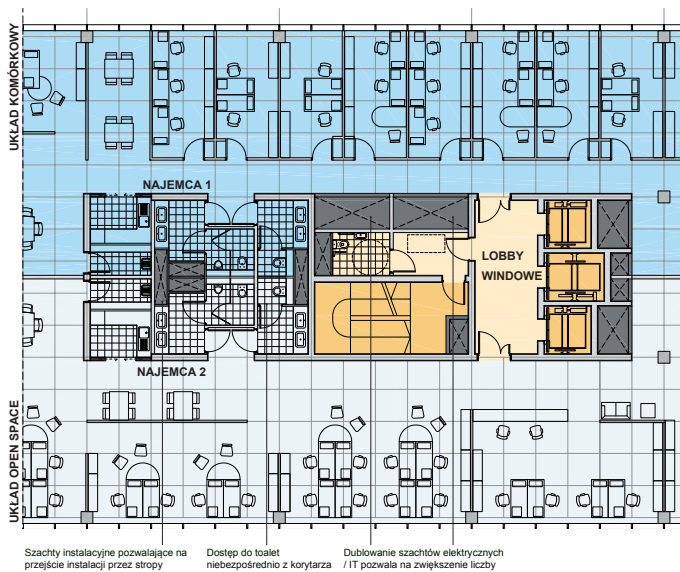
Przykład trzonu z toaletami przypisanymi poszczególnym najemcom
