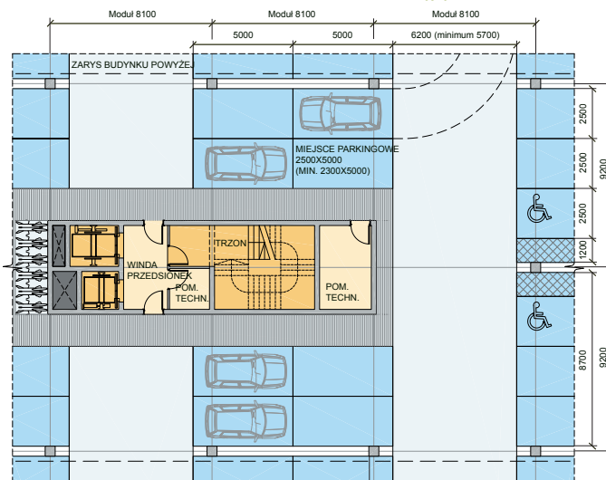
Siatka projektowa i konstrukcyjna – rzut parkingu podziemnego SŁUPY ODSUNIĘTE ABY UŁATWIĆ MANEWROWANIE
