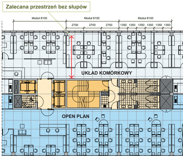
Siatka projektowa i konstrukcyjna – rzut kondygnacji biurowej Typowy rzut Siatka konstrukcyjna 8,10m Moduł ścianek działowych 2,70m Moduł elewacyjny 1,35m
