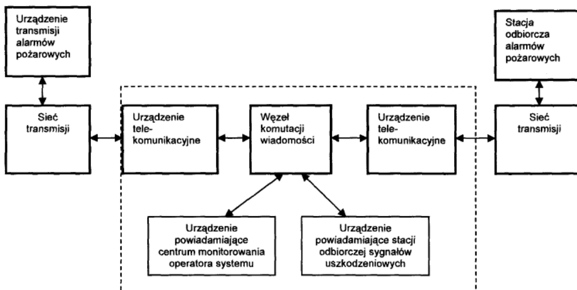
Rys. nr 10.4.2.2. Tor transmisji alarmów pożarowych poprzez centrum odbiorcze operatora systemu
