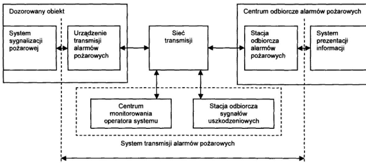
Rys. nr 10.4.2.1. Schemat systemu transmisji alarmów pożarowych
