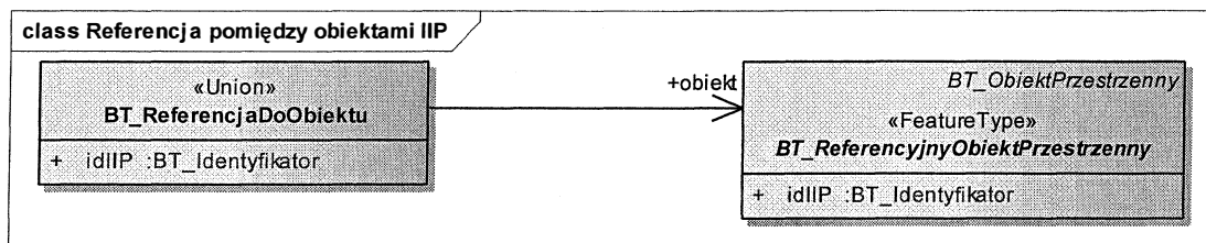
Diagram: Referencja pomiędzy obiektami IIP
