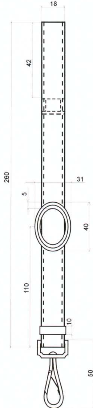
WYMIARY widok z przodu
